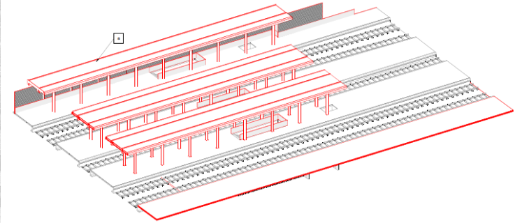
Spaccato Assonometrico
